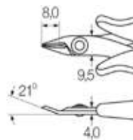
meget smalt, spidst hoved uden skrå kant
